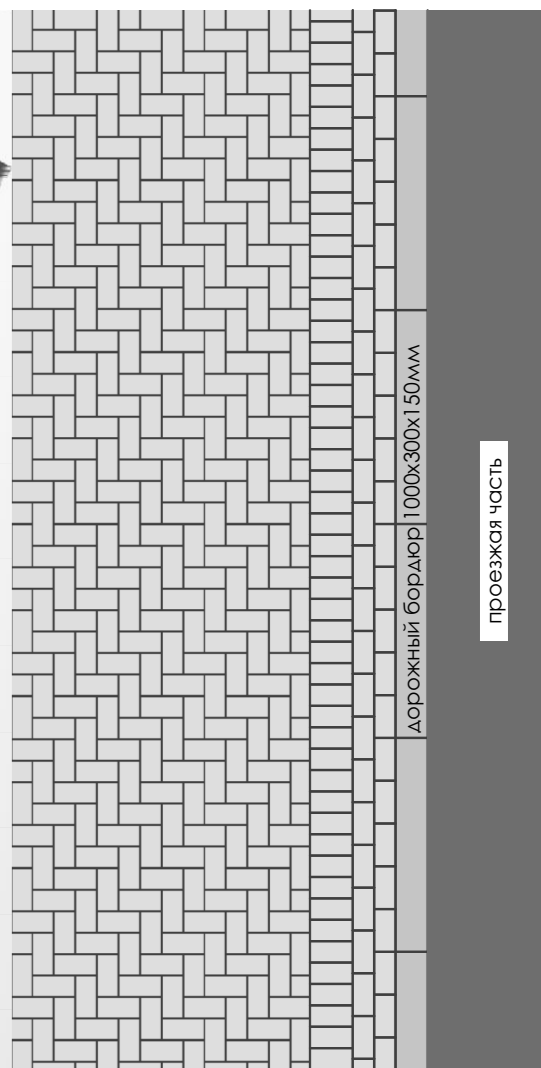
фрагмент мощения тротуара
